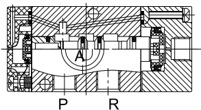
单气控(常开)
