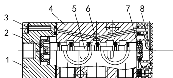
单气控
