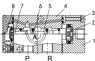
单气控(常闭)
